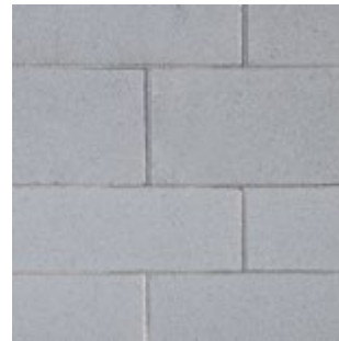
BETONPFLASTER MANHATTAN betonglatter Betonstein, Hellgrau, hydrophobiert, Formatmix im Reihenverband, 18 Steine pro Lage Stärke: 80 mm (EAN 4333990719185)
